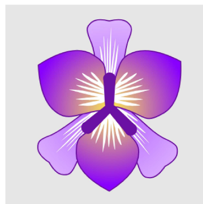
Iris Virginica
